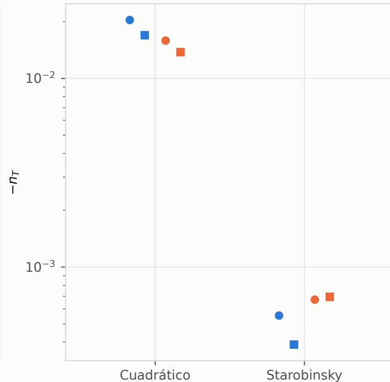
(b) Índice tensorial (azul RG, naranja UG)
