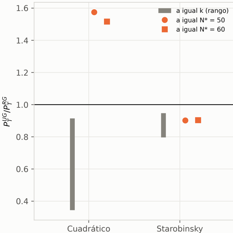
(a) Cociente de P_T (UG/RG)
