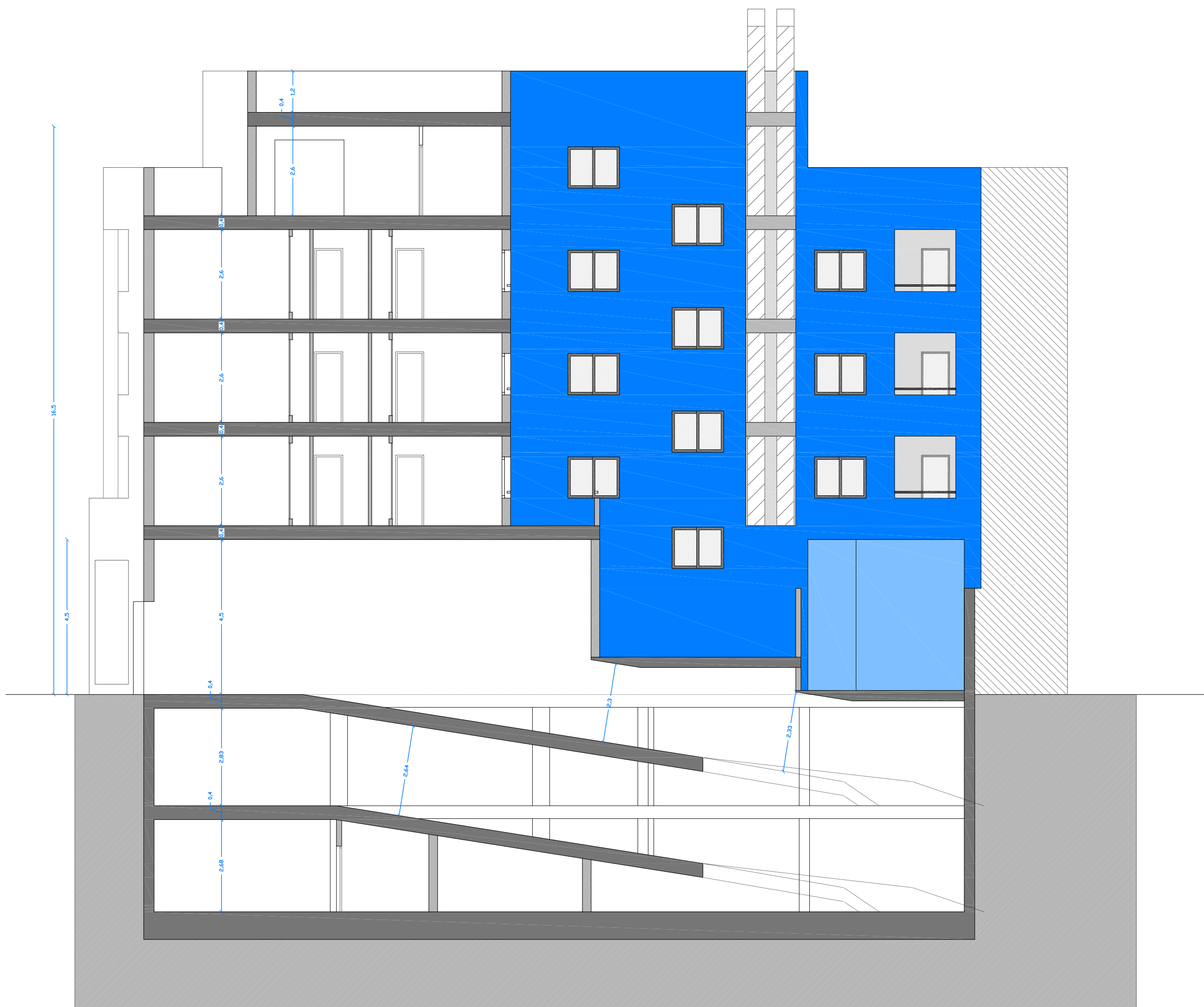
SECCION LONGITUDINAL L1-L1' E/1:100
