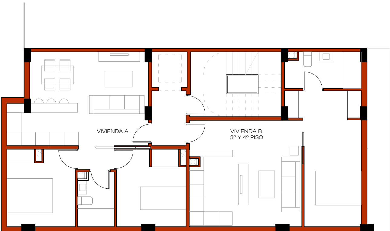
PLANTA 3º-4º
