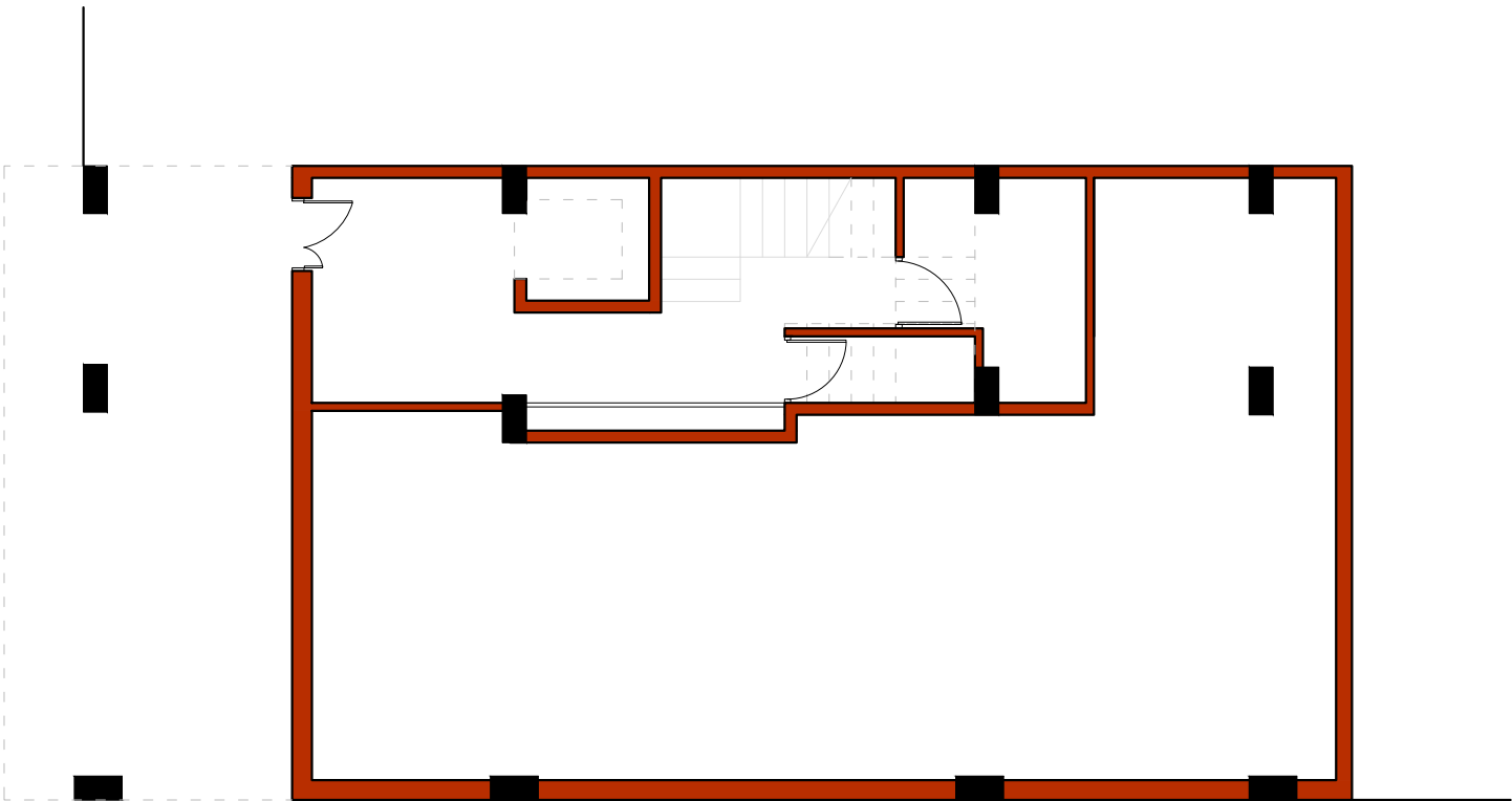
PLANTA BAJA
