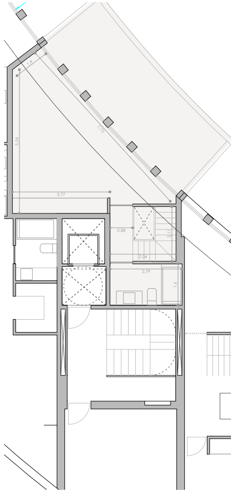
Planta Bajo Cubierta
