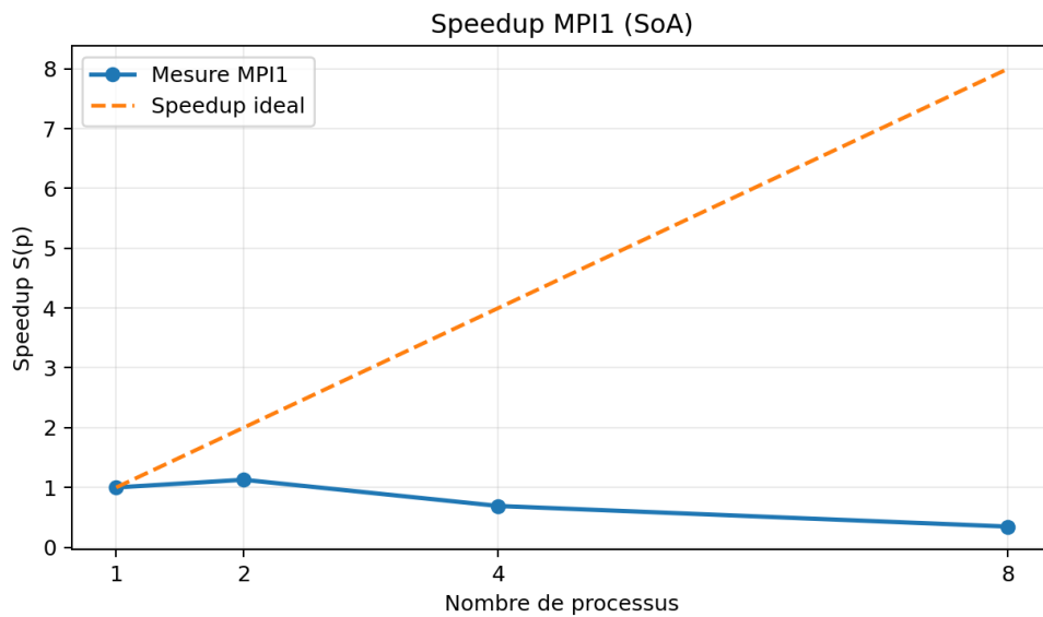
FIGURE 5 – Speedup mesuré MPI1 (SoA) pour K = 1 vs speedup idéal linéaire
