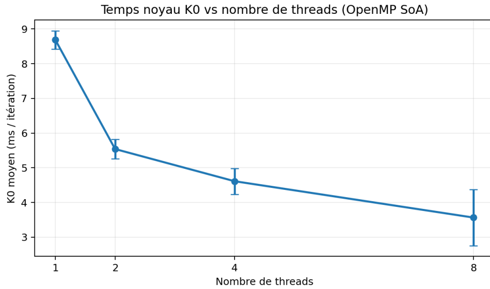
FIGURE 3 – Temps noyau K0 en fonction du nombre de threads (barres d'erreur : écart-type)
