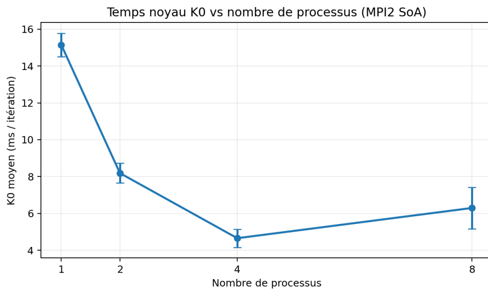
FIGURE 13 – Temps noyau K0 en fonction du nombre de processus (MPI2 SoA)
