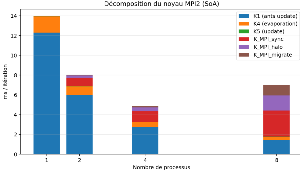
FIGURE 14 – Décomposition K1/K4/K5/K_{\text{MPI\_sync}}/K_{\text{MPI\_halo}}/K_{\text{MPI\_migrate}}
