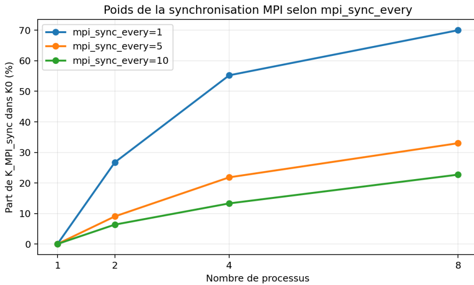
FIGURE 10 – Part de K_{\text{MPI\_sync}} dans K_0 selon mpi_sync_every
