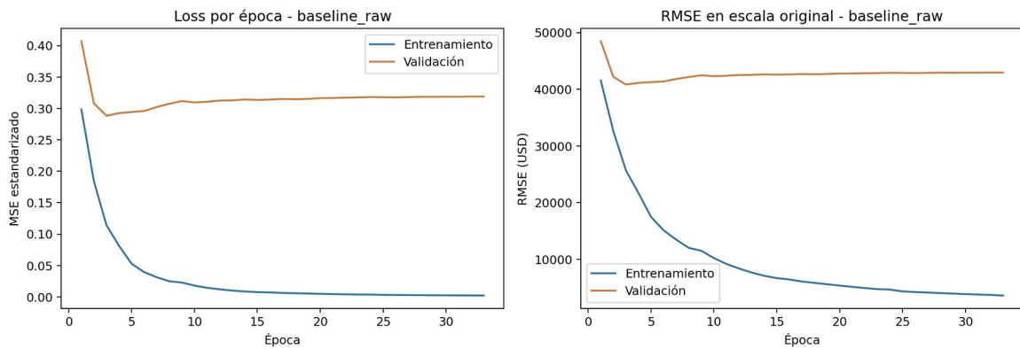
Figura 5. Loss y RMSE de entrenamiento/validación del MLP baseline.
