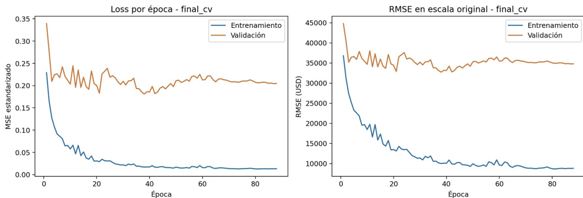
Figura 6. Loss y RMSE de entrenamiento/validación del modelo ganador en CV.
