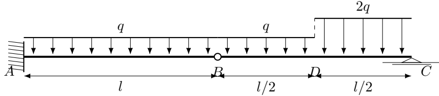
图 3: 连片组合梁的受力与尺寸图
