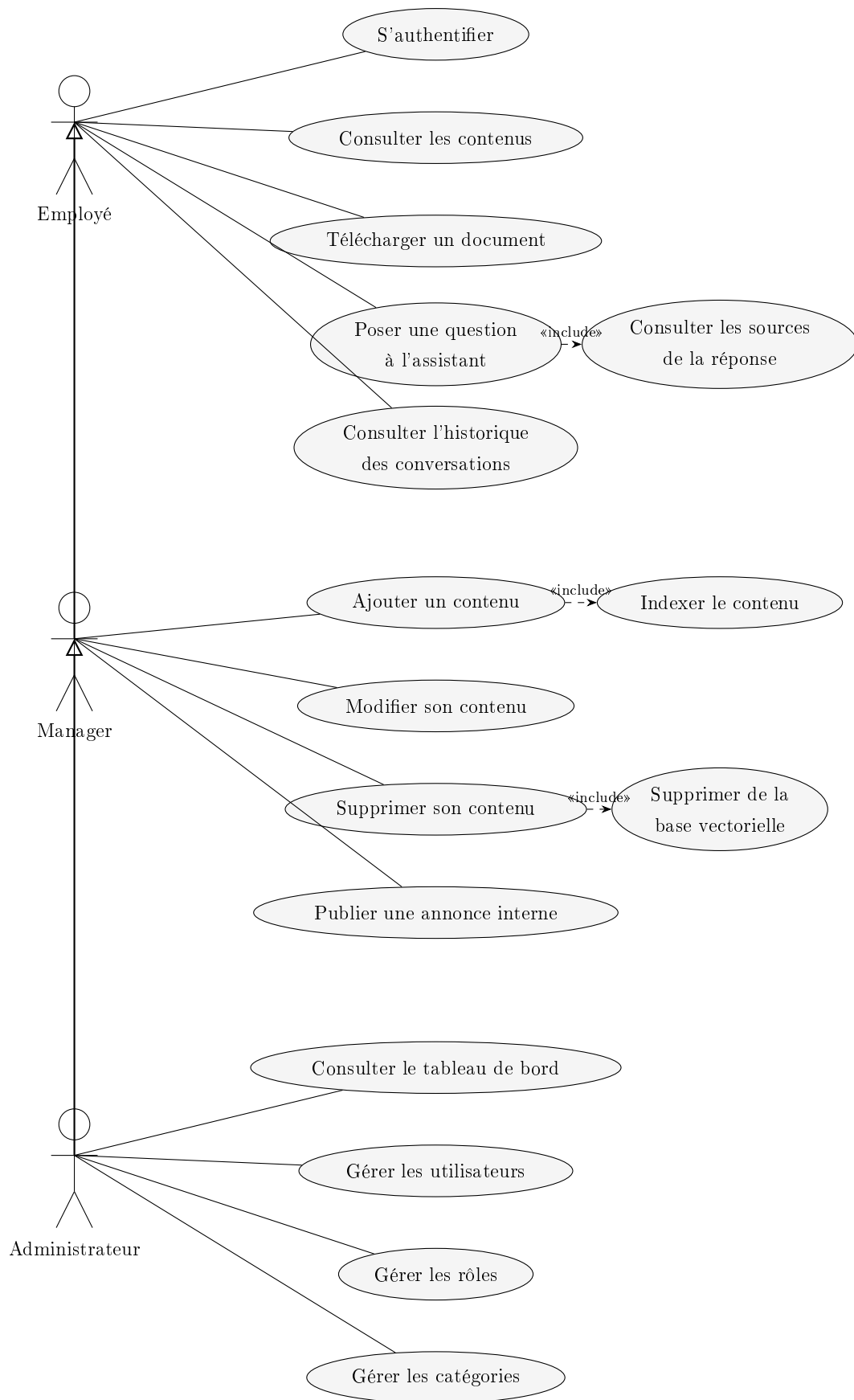
Figure 2.4: Diagramme de cas d'utilisation (avec généralisation des acteurs)
