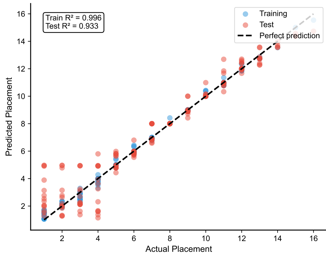
Predicted vs Actual Placement
