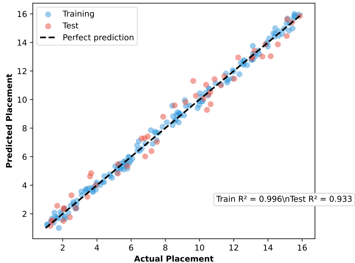
Predicted vs Actual Placement
