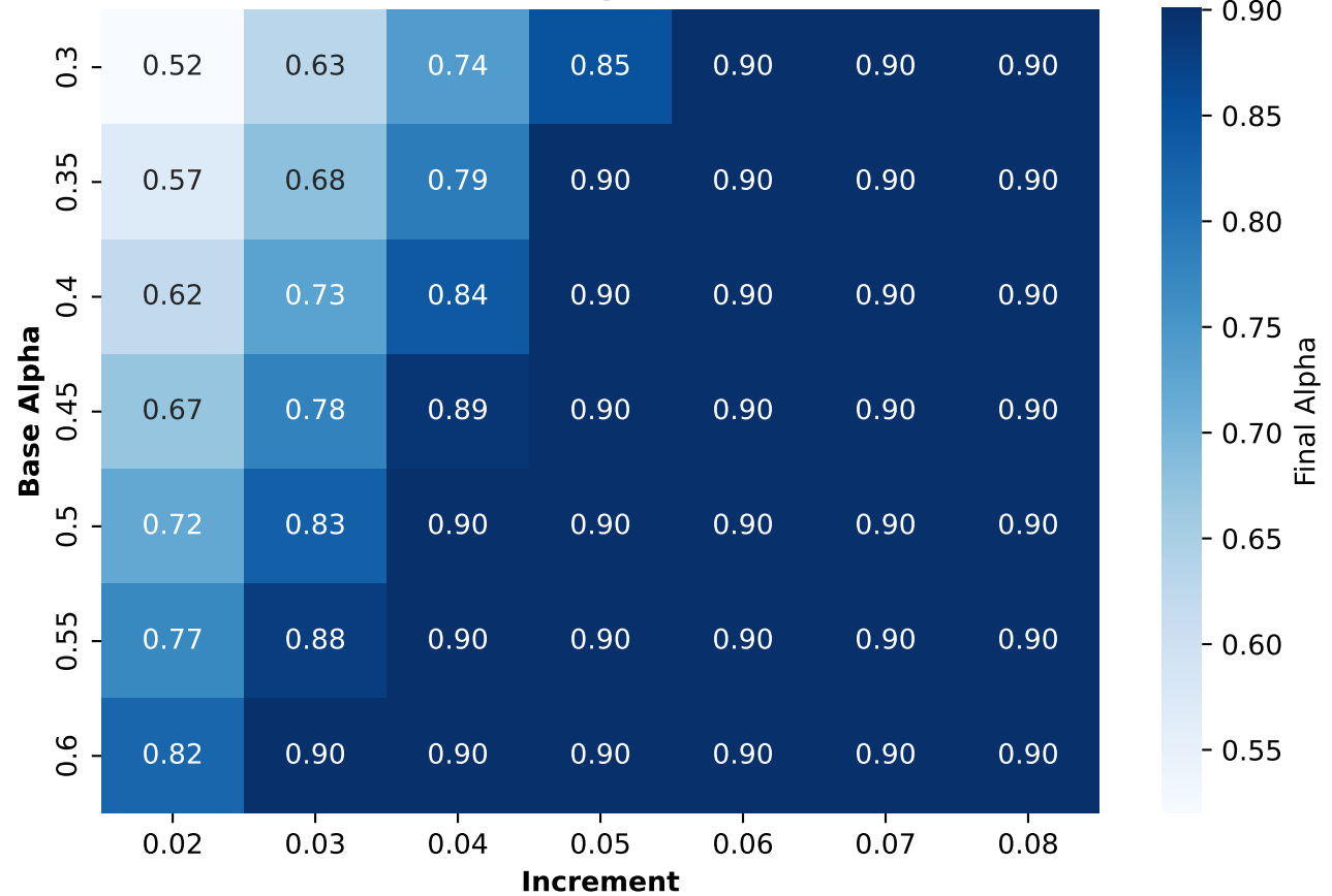
(b) Final Alpha Values
