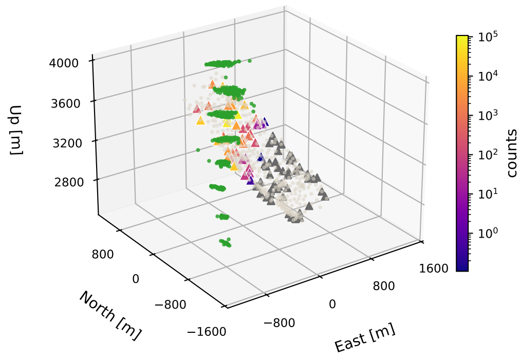
#64 (Elow/vert) E=3.5e+05, \theta=78^\circ , \phi=59^\circ , 50/100
