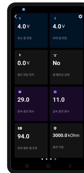
서브 배터리 (EV) 셀 전압·절연저항
