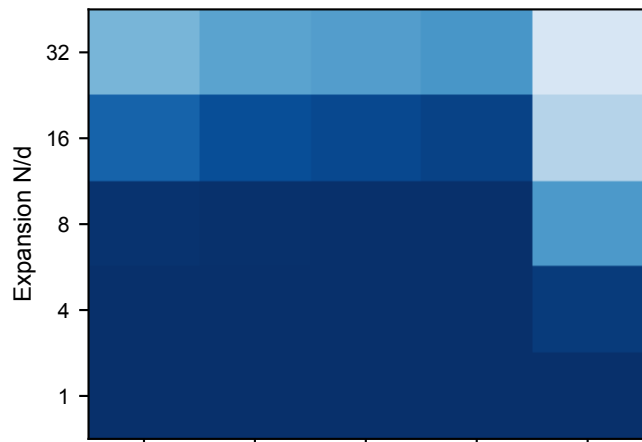
ECG-JEPA
