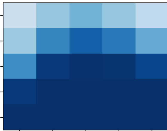
HuBERT-ECG
