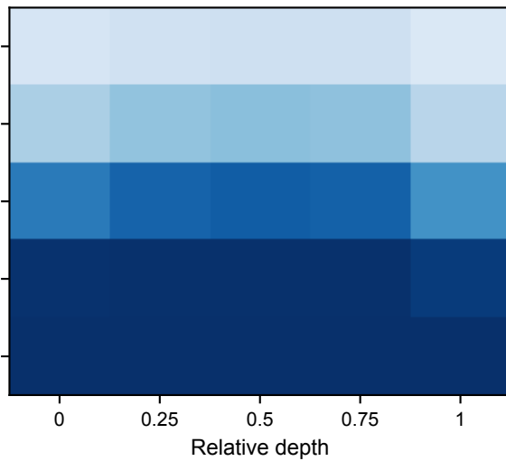
HuBERT-ECG
