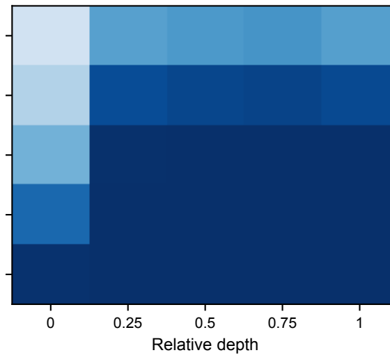
ST-MEM
