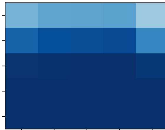
ST-MEM
