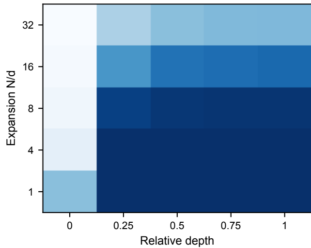
ECG-JEPA
