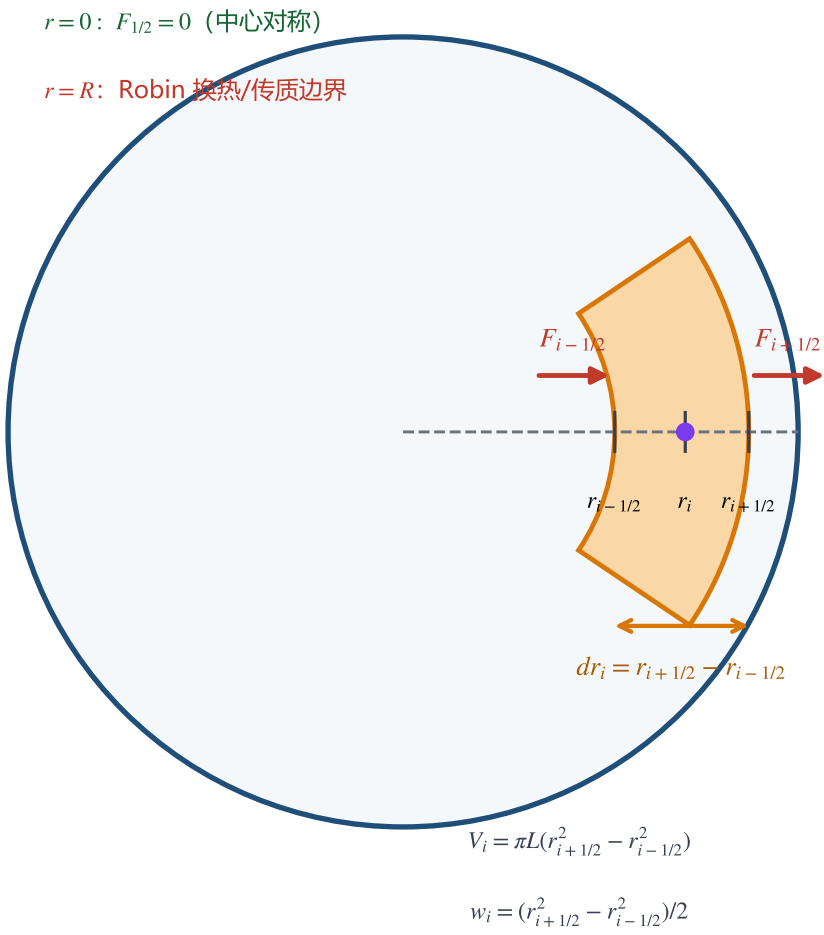
(b) 环形控制体与 dr
