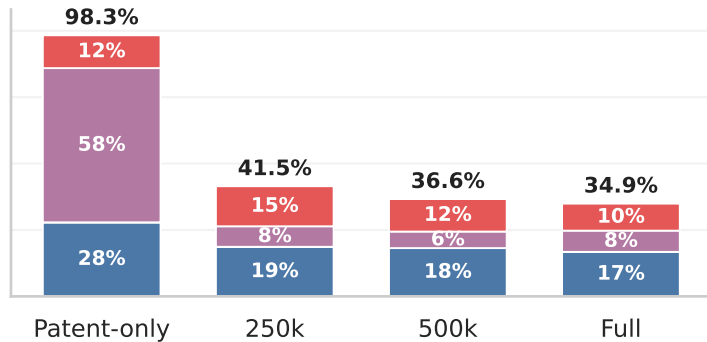
TabSyn
