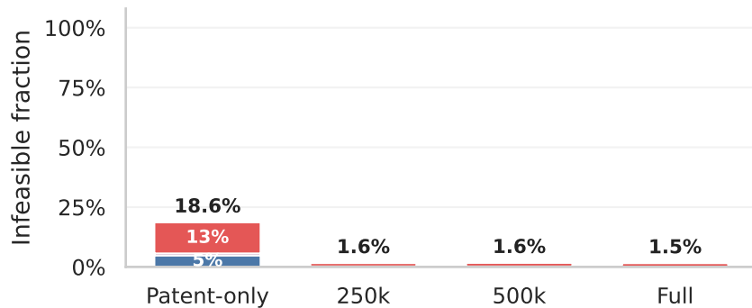
TabDDPM
