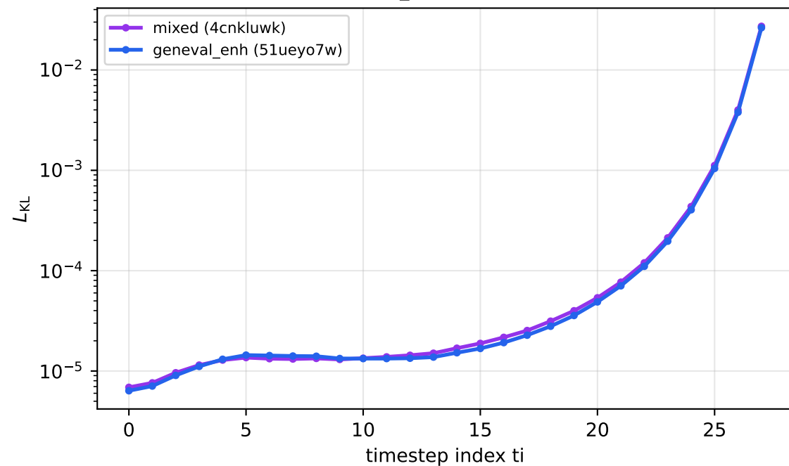
mean_tail L_{KL} (conv.)
