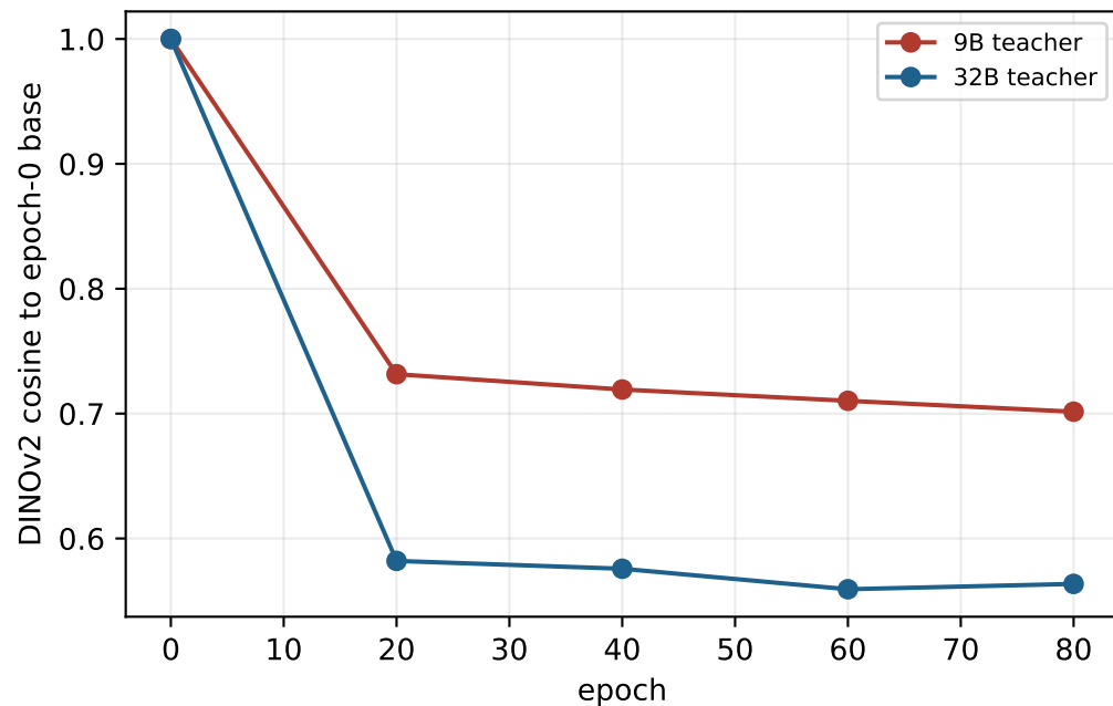
(d) Same-seed arms separate after epoch 0
