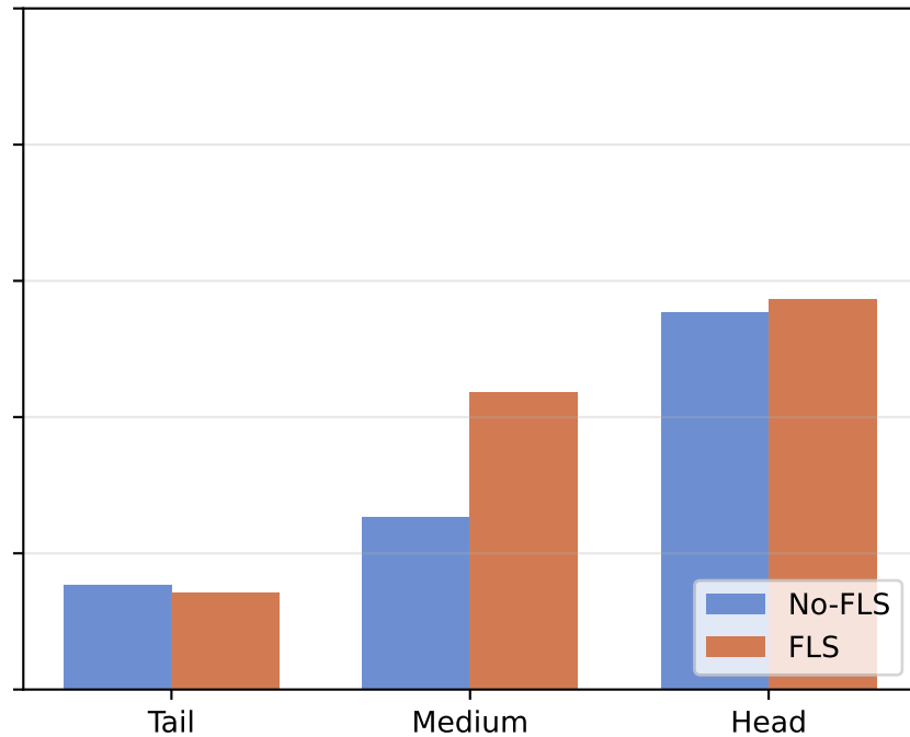
Macro F1
