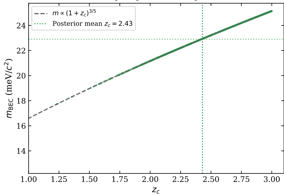
BEC mass vs condensation redshift (Step 10 posterior samples)
