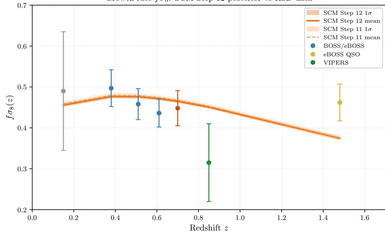
Growth rate f\sigma_8 : SCM Step 12 posterior vs RSD data
