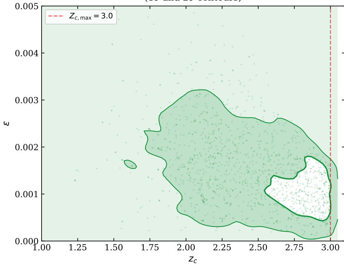
Step 10: \varepsilon vs z_c posterior ( 1\sigma and 2\sigma contours)
