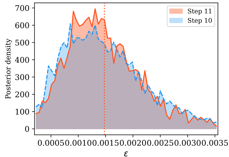
Step 10 vs Step 11 Posterior Comparison
