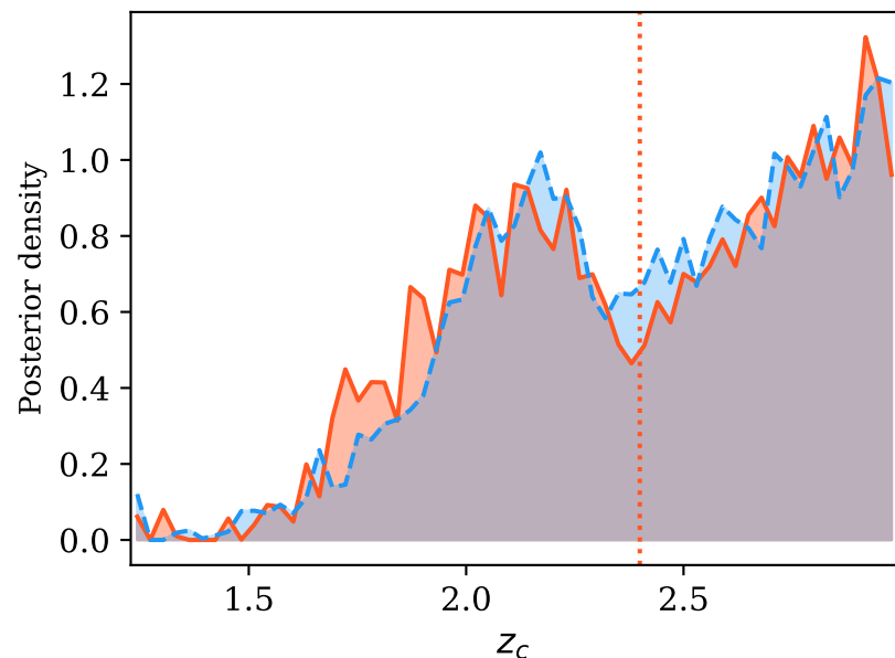
Step 10 vs Step 11 Posterior Comparison
