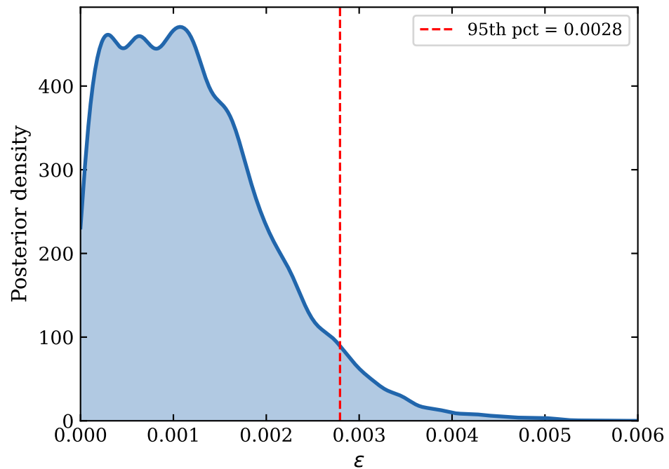
Step 7: \varepsilon posterior ( \varepsilon < 0.0028 at 95\%)
