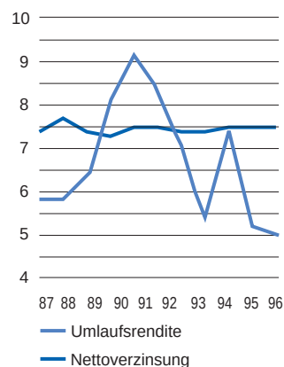
Nettoverzinsung und Umlaufrendite in Prozent
