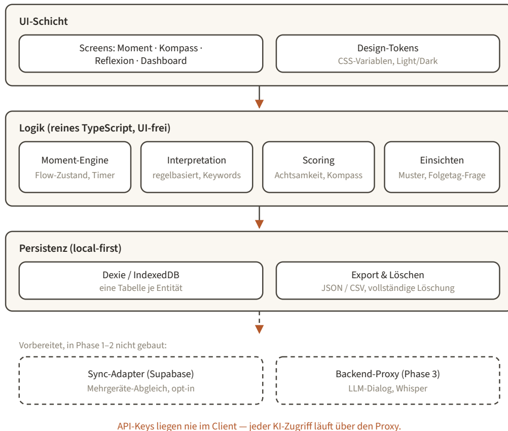
Abb. 10.1 — Schichtenarchitektur: local-first Kern, gestrichelt die vorbereiteten Phase-3-Erweiterungen.
