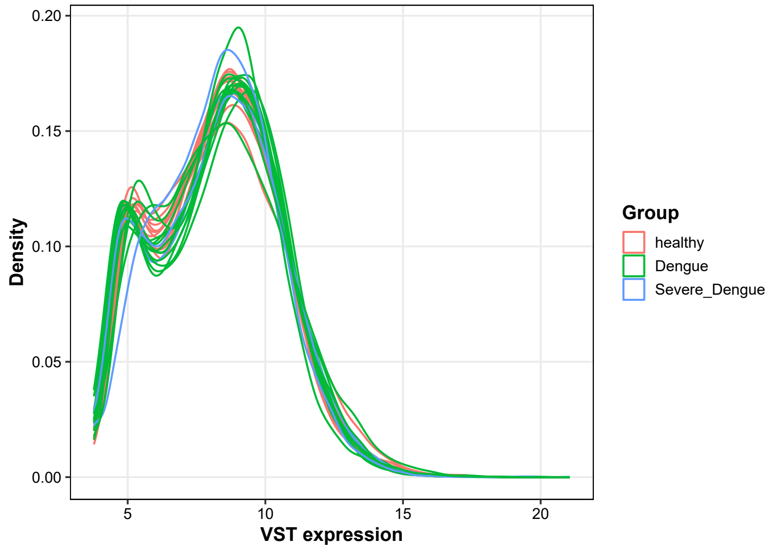
VST density plot
