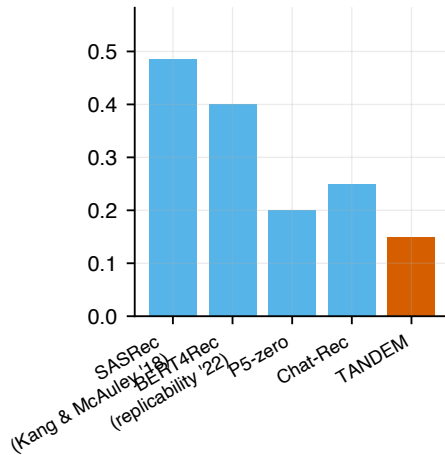
Hit@10
