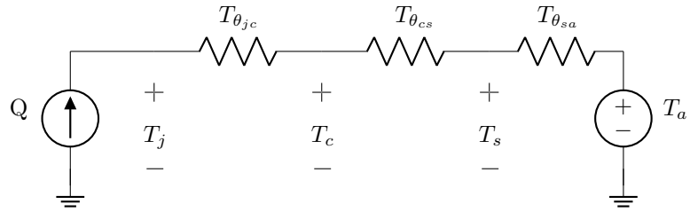
Figura 1: Circuito Térmico equivalente con disipador.
