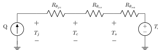
Figura 4: Circuito térmico equivalente con disipador.
