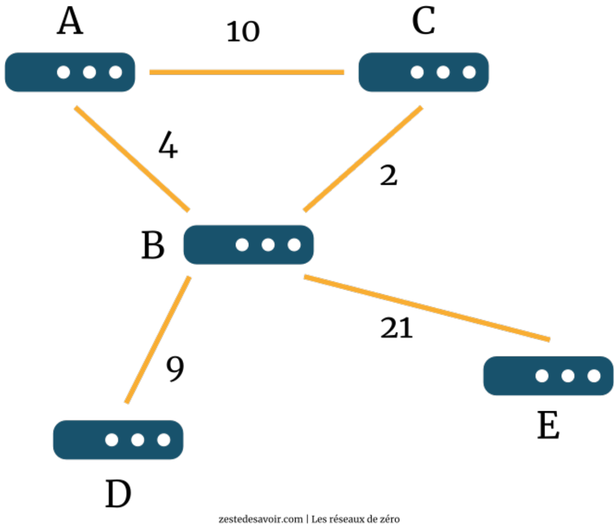
FIGURE IV.7.3. – Interconnexion de 5 routeurs avec des sauts entre chaque (CC BY)
