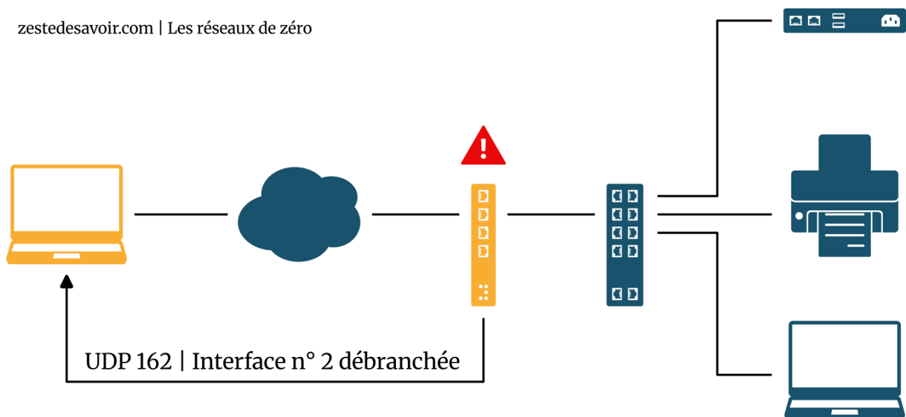
FIGURE VI.5.4. – Le trap SNMP permet à un agent d'informer immédiatement le superviseur d'un évènement (CC BY)
