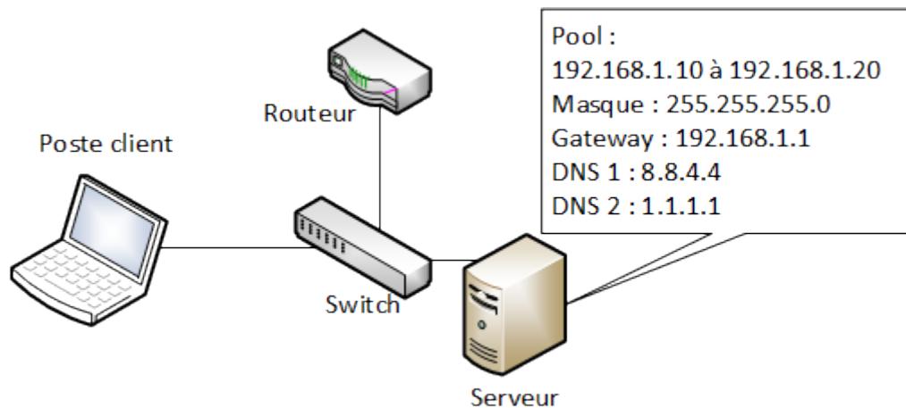
FIGURE VI.2.7. – Ce que "voit" un serveur DHCP
