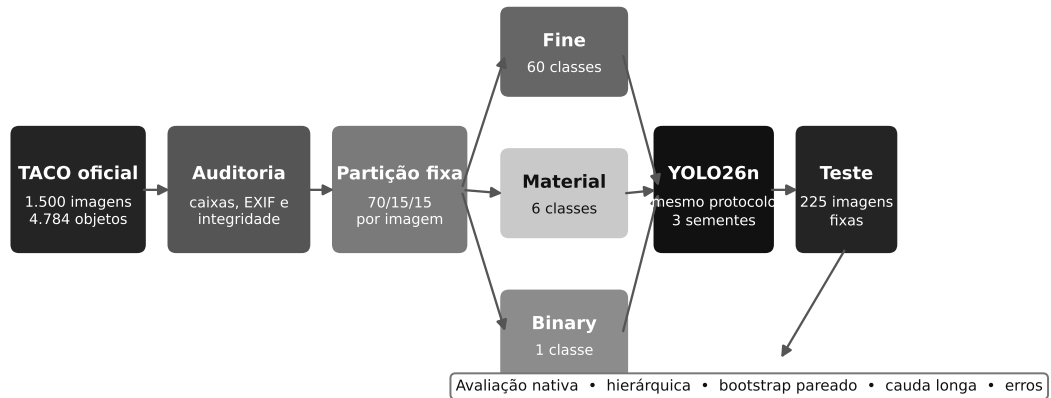
Figura 1. Pipeline experimental. Somente a taxonomia varia entre os três ramos de treinamento; imagens, caixas, partição, arquitetura e hiperparâmetros permanecem fixos.
