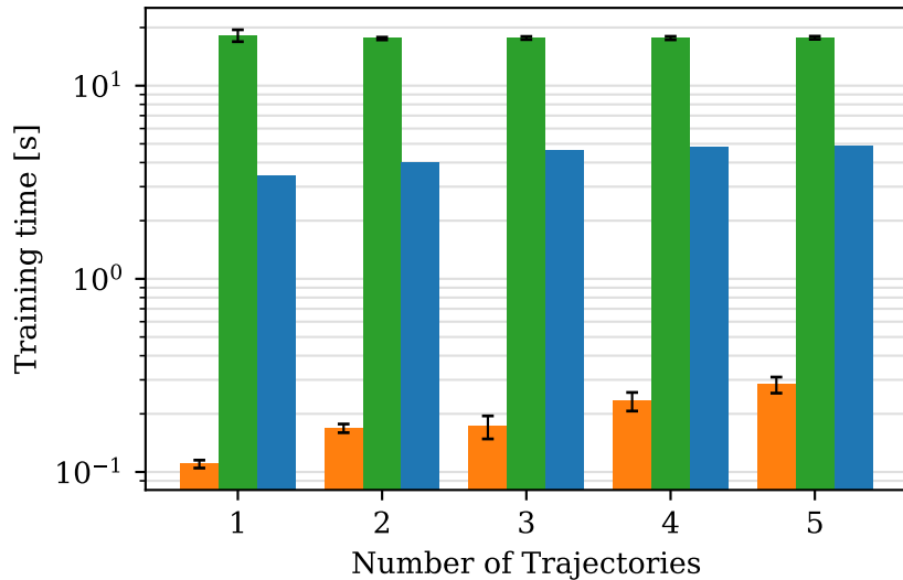
Spring-mass
