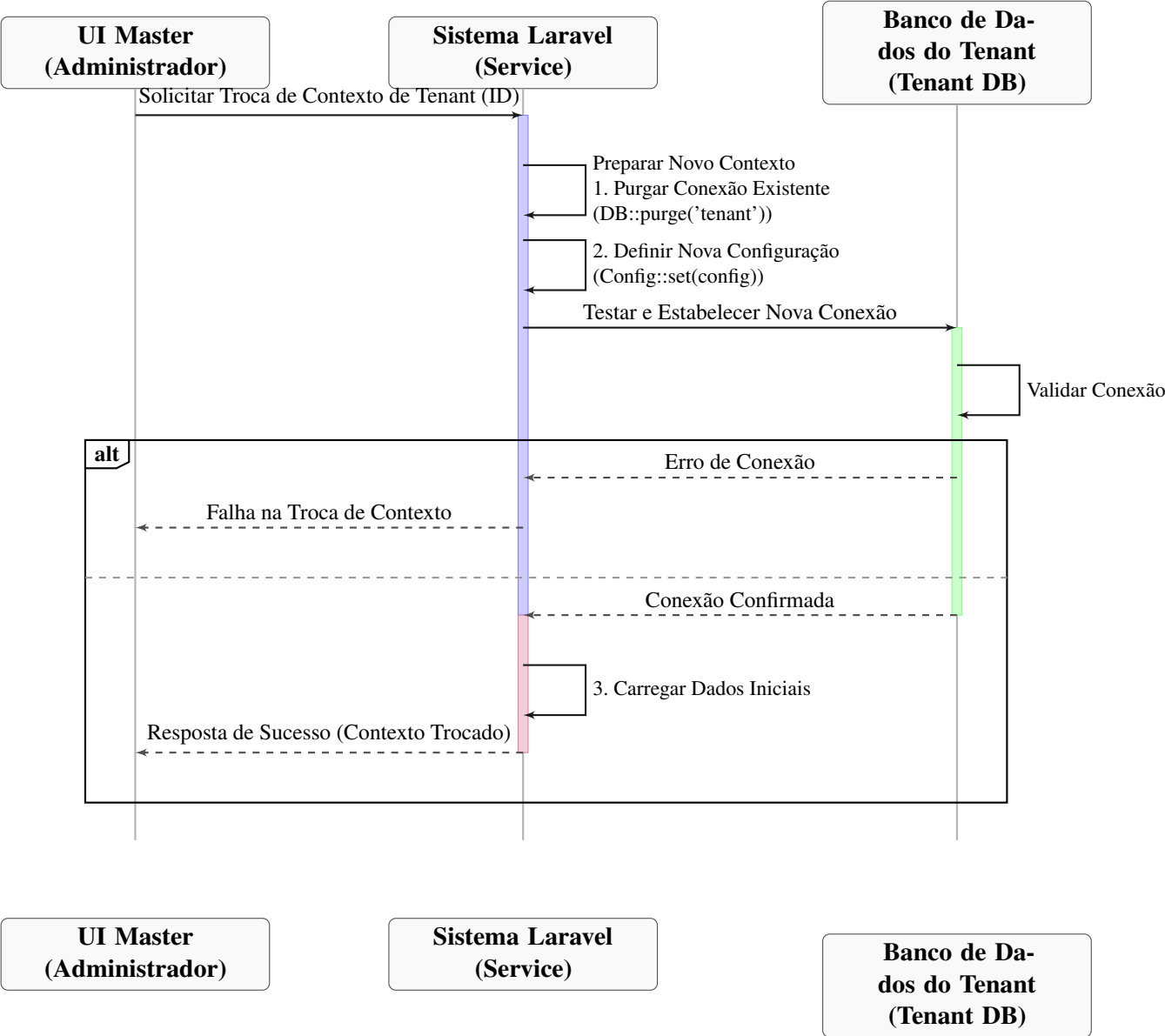
Figura 5 – Diagrama de Sequência: Alternância Dinâmica de Contexto de Tenant ( Tenant Switcher )
