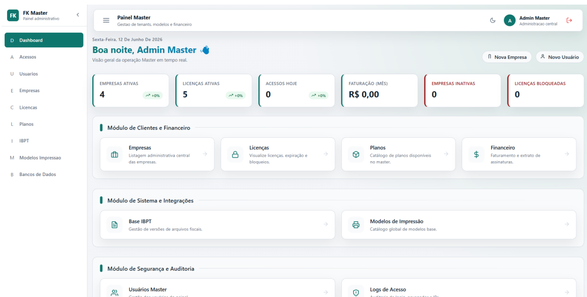
Figura 6 – Dashboard Administrativo: Painel Integrado de KPIs e Telemetria
