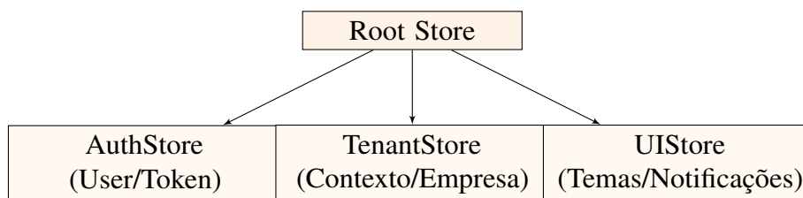
Figura 16 – Organização das Stores Globais (Pinia)
