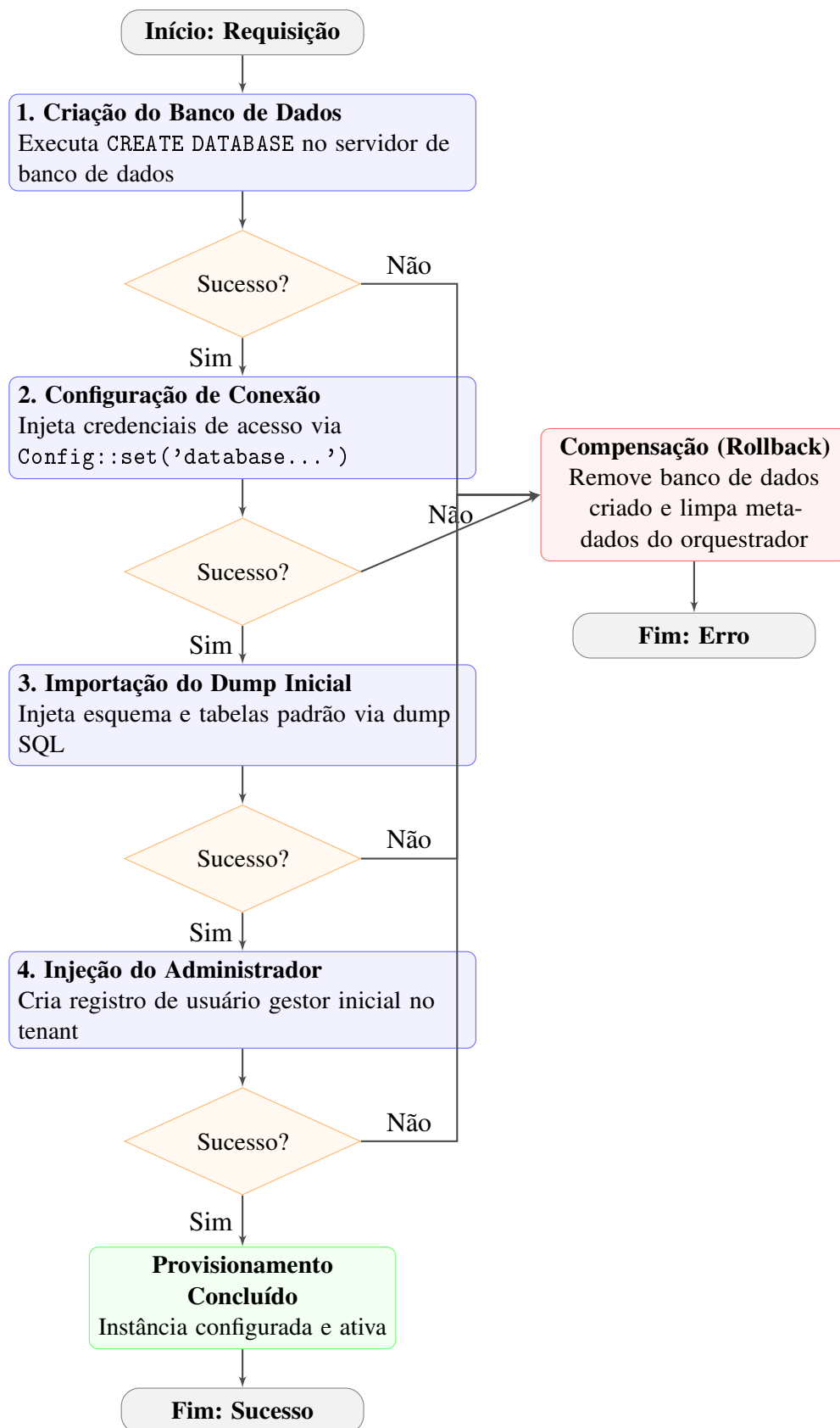
Figura 4 – Diagrama de Atividades: Provisionamento Automatizado de Nova Instância
