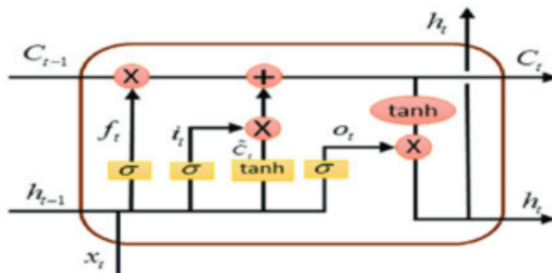
Figura 2.5: Arquitectura LSTM
