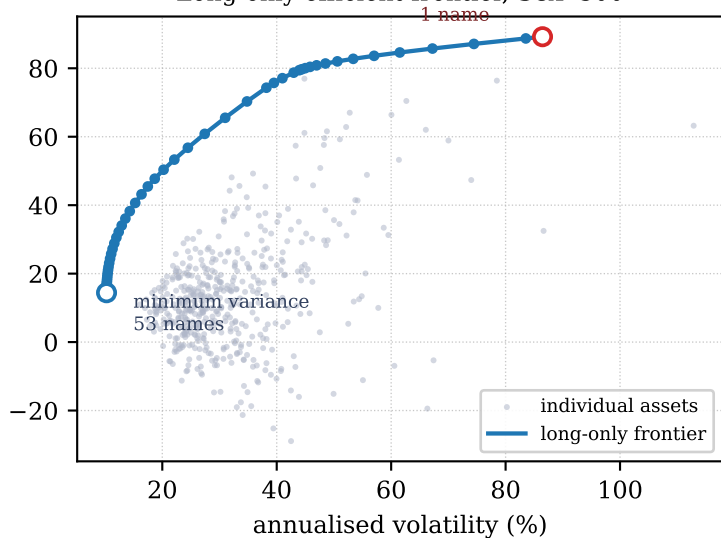
Long-only efficient frontier, S&P 500
