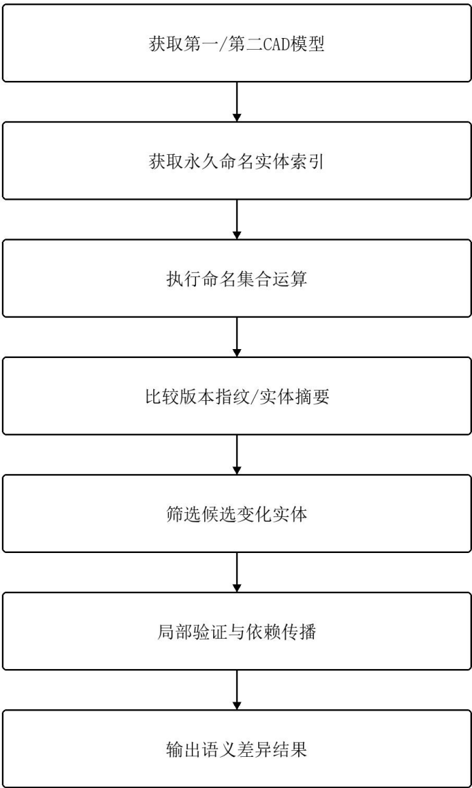
图1 基于永久命名的CAD模型差异对比方法流程图
