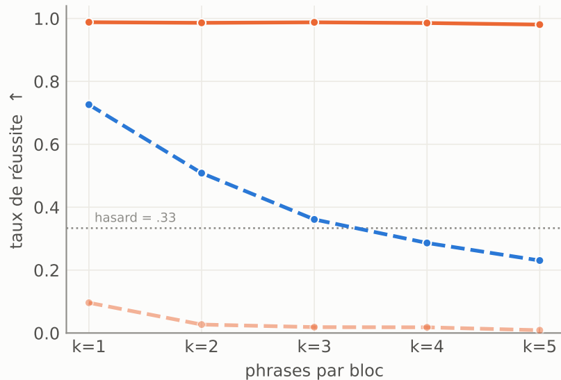
Taux de réussite, D = 2 distracteurs
