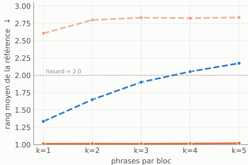
Rang moyen, D = 2 distracteurs
