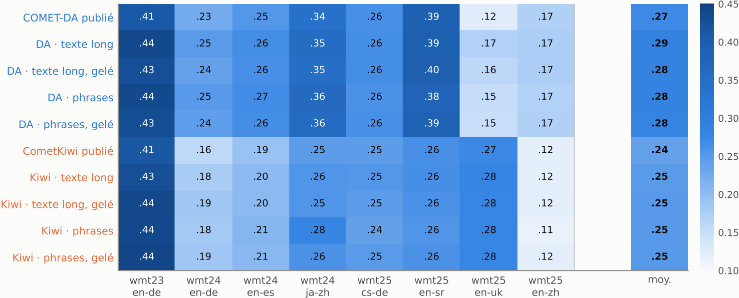
Documents natifs — Kendall \tau par jeu de test
