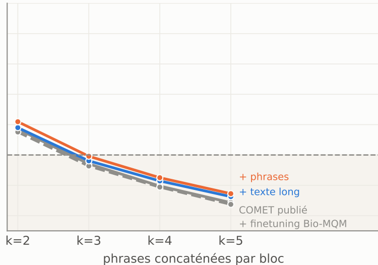
Variantes de l'encodeur COMET (même échelle)
