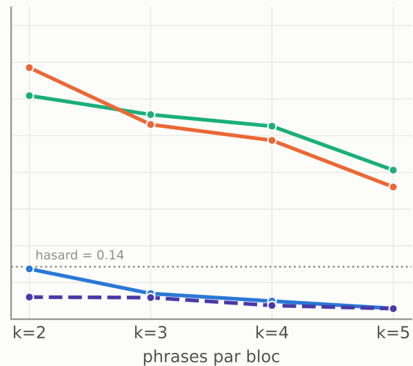
D = 6 distracteurs
