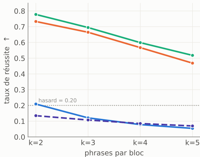
D = 4 distracteurs
