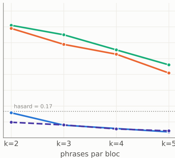
D = 5 distracteurs
