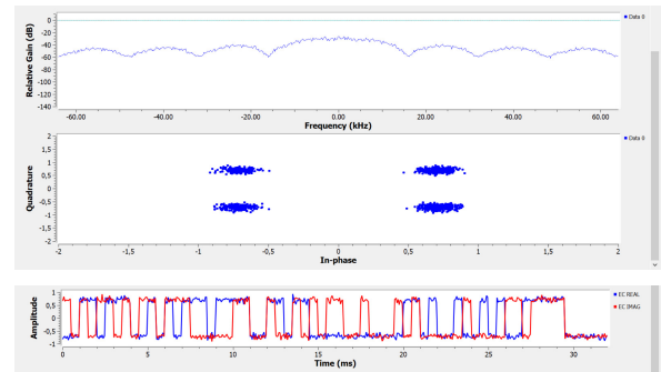
Figura 7: Análisis de señales para modulación QPSK: componentes en fase y cuadratura, PSD y diagrama de constelación con M = 4 .
