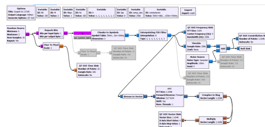
Figura 1: Diagrama de bloques general para la implementación del transmisor M-PSK en GNU Radio.
