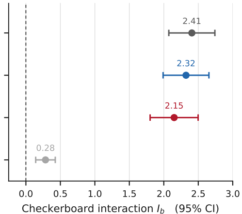
(b) Gemma-2-9B-it, layer 27
