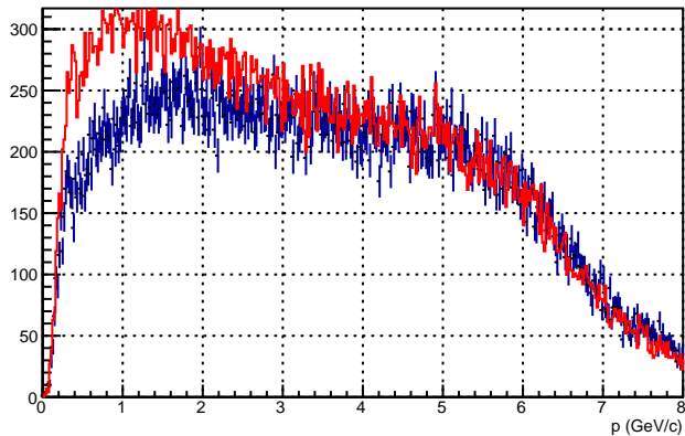
\pi^-, \gamma p \rightarrow \pi^+ \pi^- \eta p
