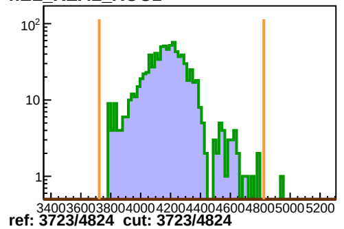
pPRE100_ROC1
