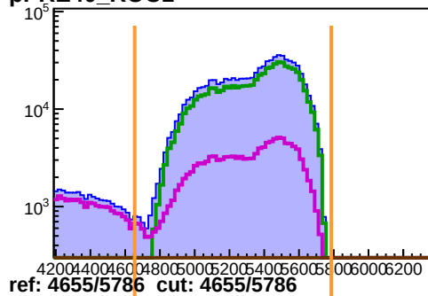
pPRE40_ROC1
