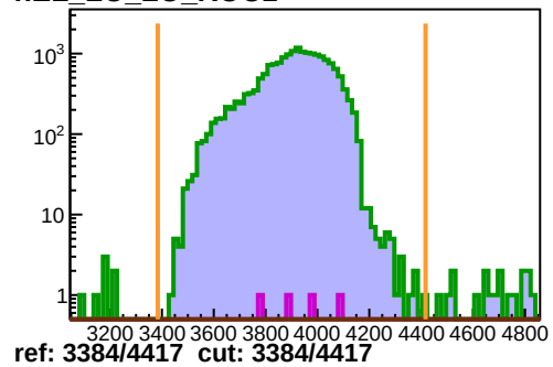
hEL_REAL_ROC1
