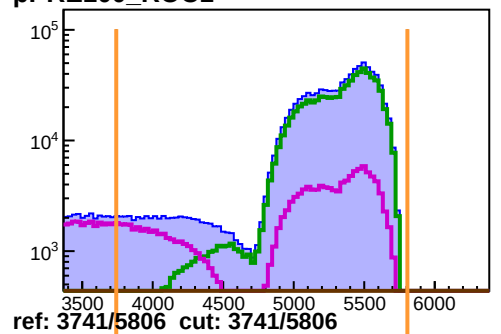
pPRE100_ROC1
