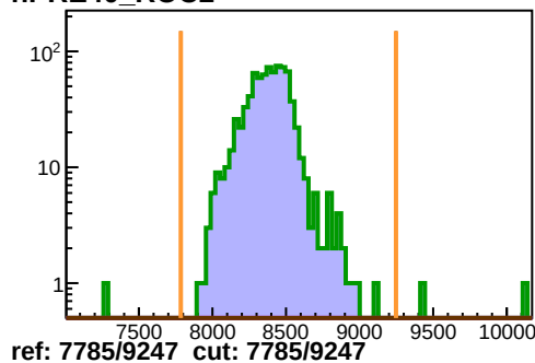
hPRE40_ROC2
