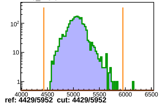
hPRE200_ROC1
