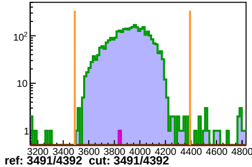
pPRE40_ROC1
