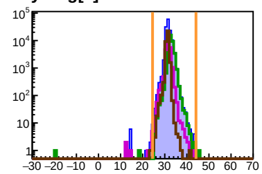
h.2y.Neg[9]
