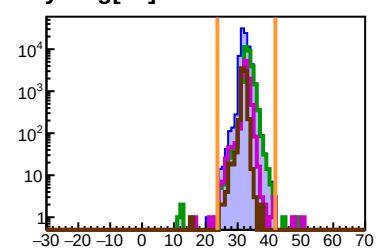
h.2y.Neg[10]
