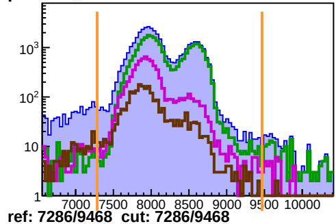
pHODO_RF
